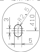
■ 据付穴詳細図
