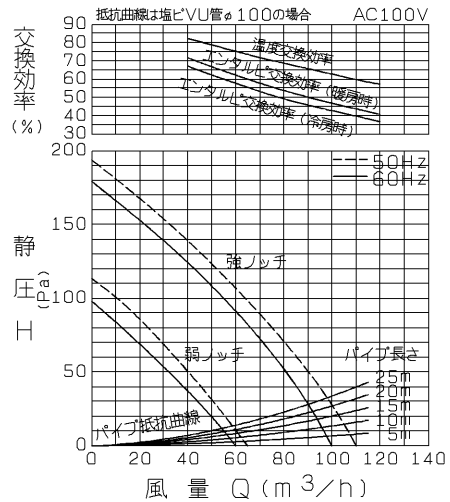
Q-H特性
