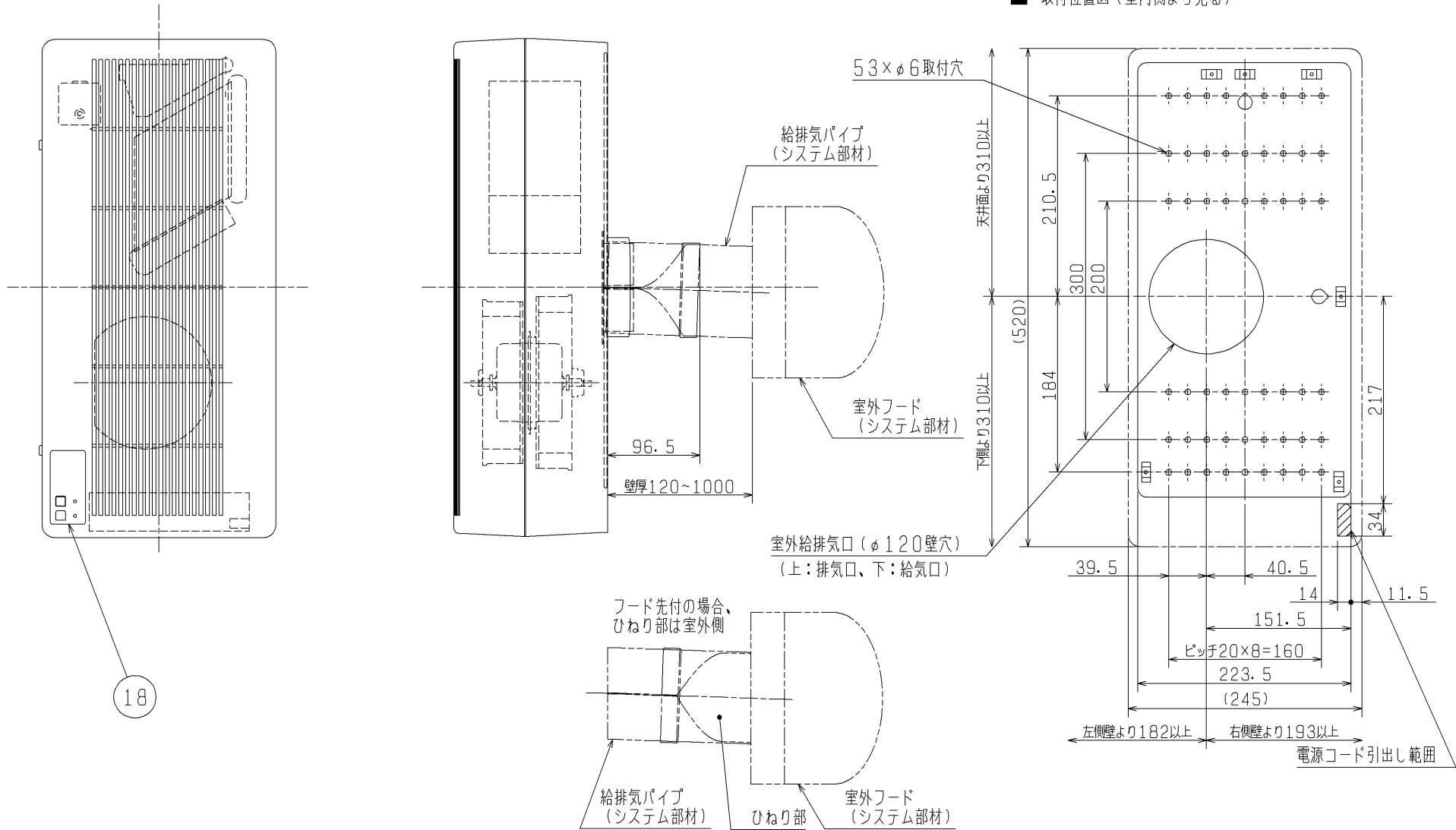
■ 取付位置図（室内側より見る）
