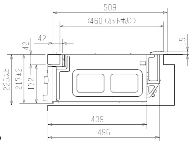
【背面図】
