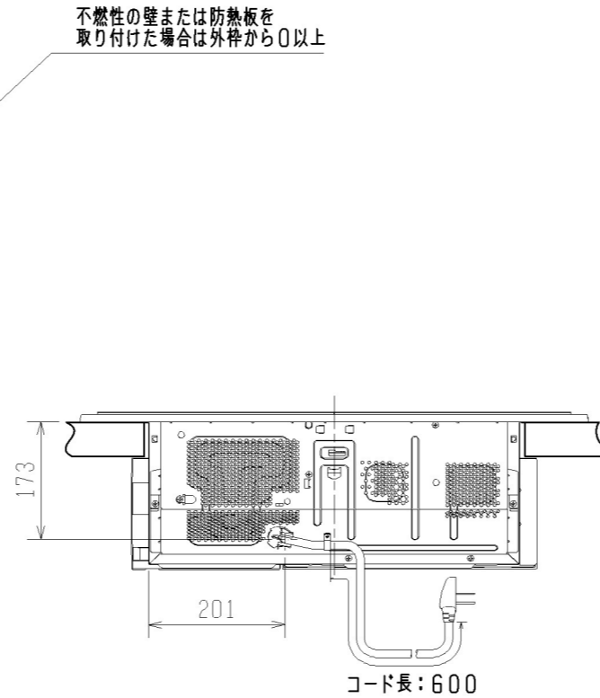
【背面図】
