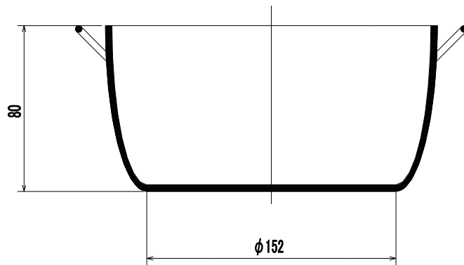
【鍋底及び側面の寸法説明図】
