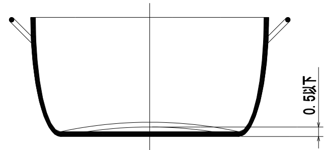
【鍋底ノ湾曲量説明図】
