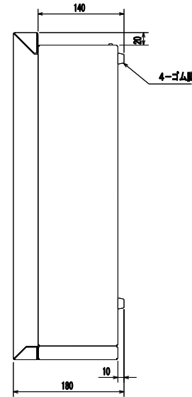
【側面図】
