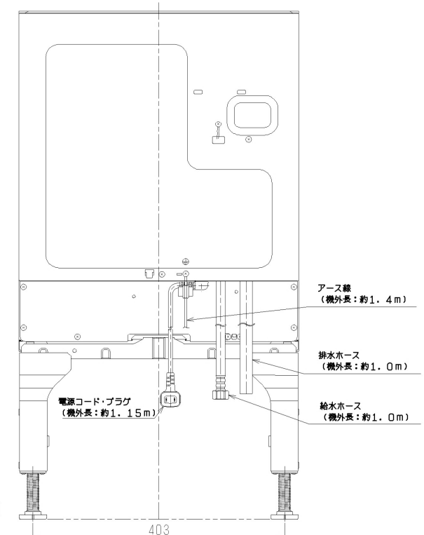
【背面図】
