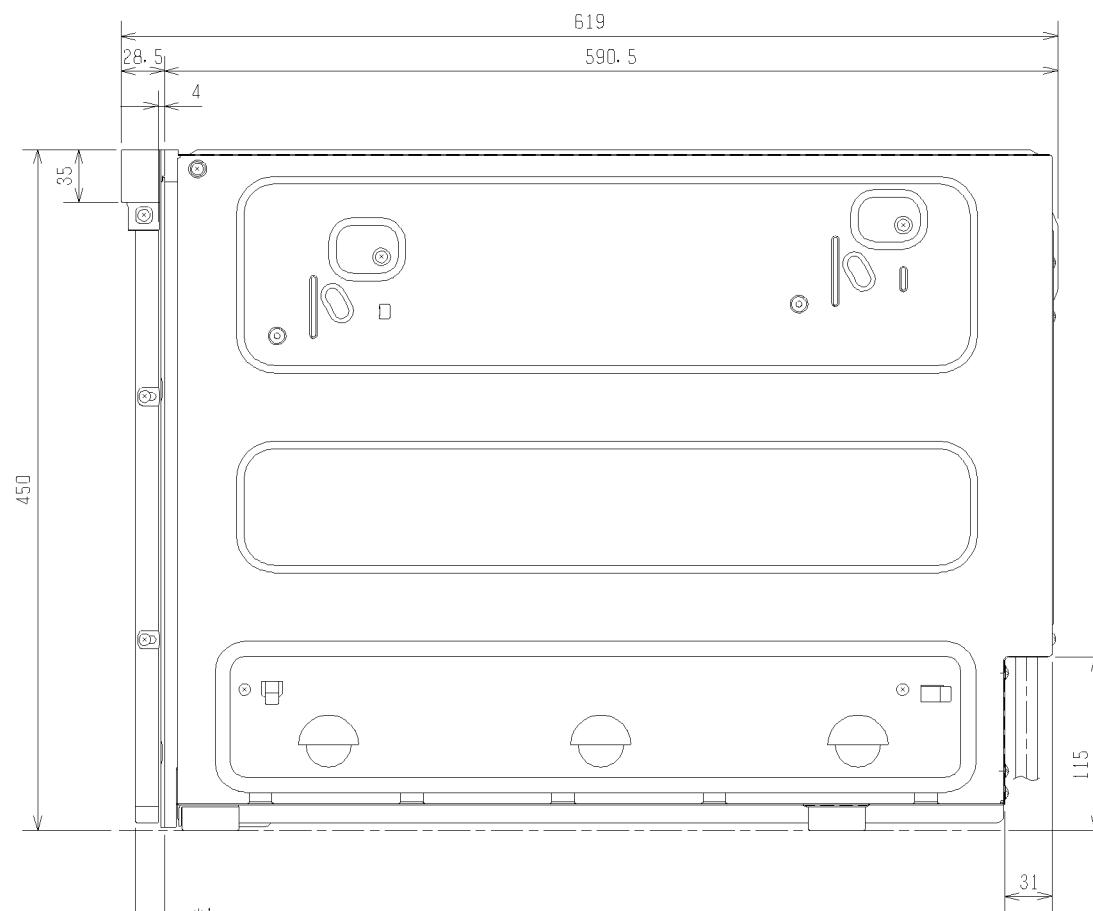
【側面図】
