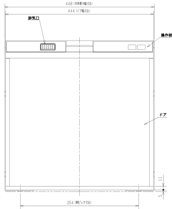
【正面図】
