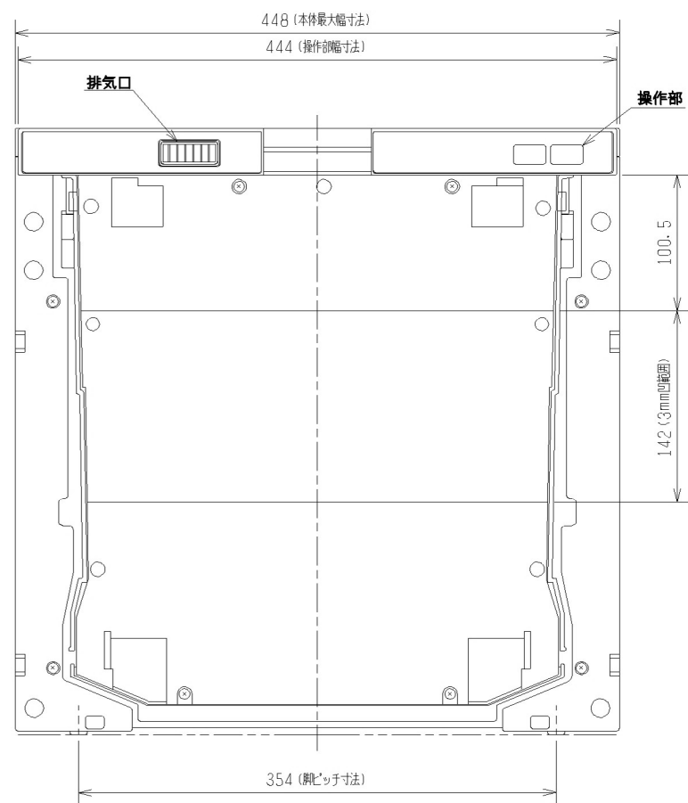
【正面図】
