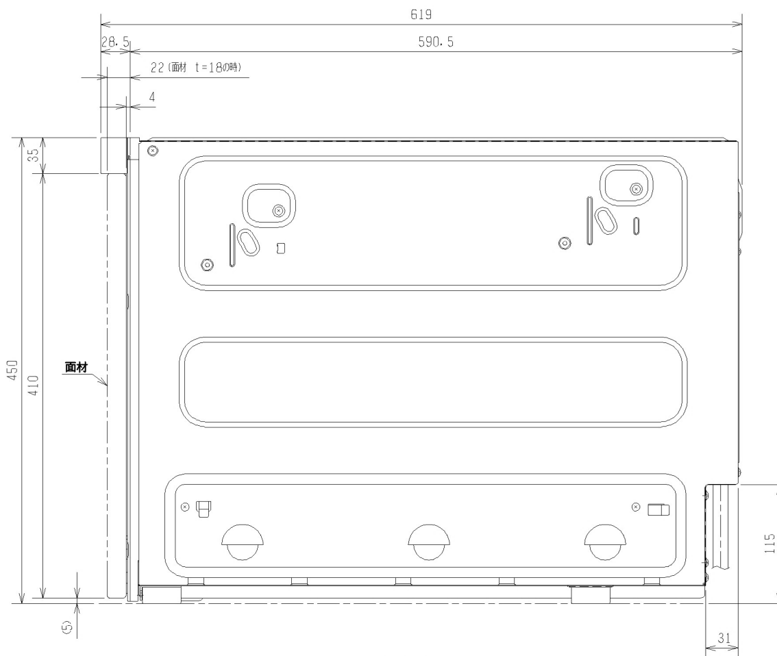
【側面図】
