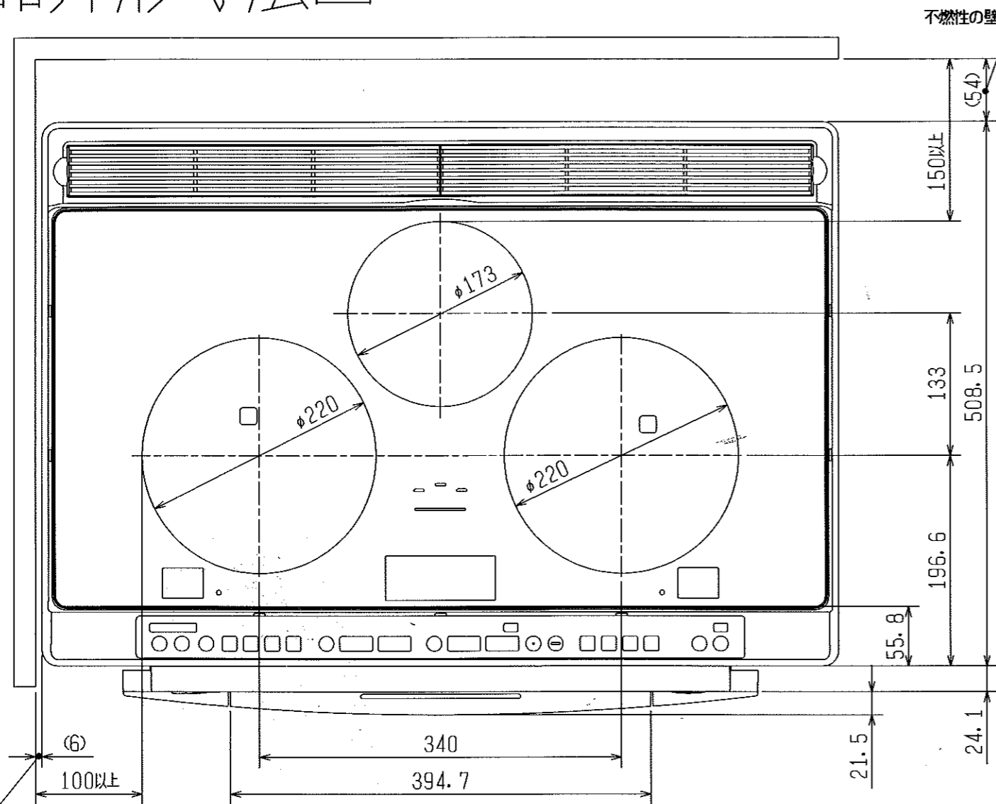
【上面図】
