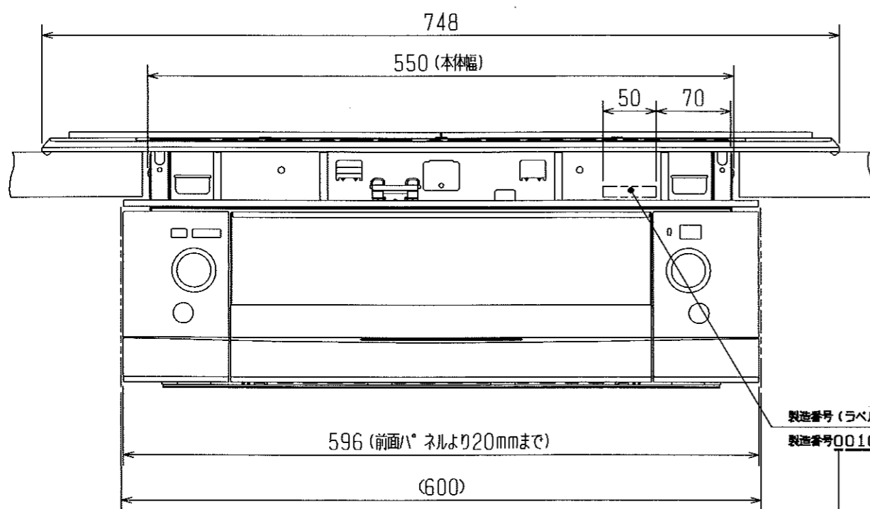
【正面図】
