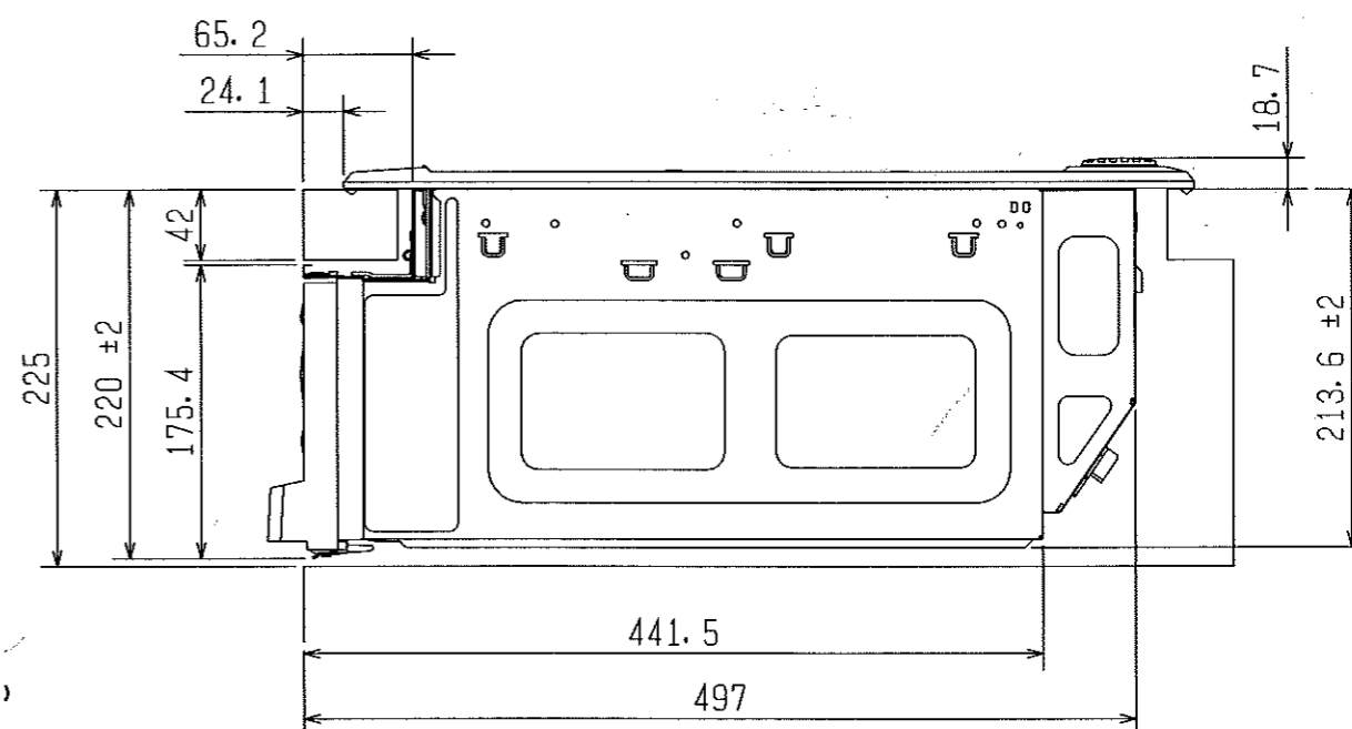
【側面図】
