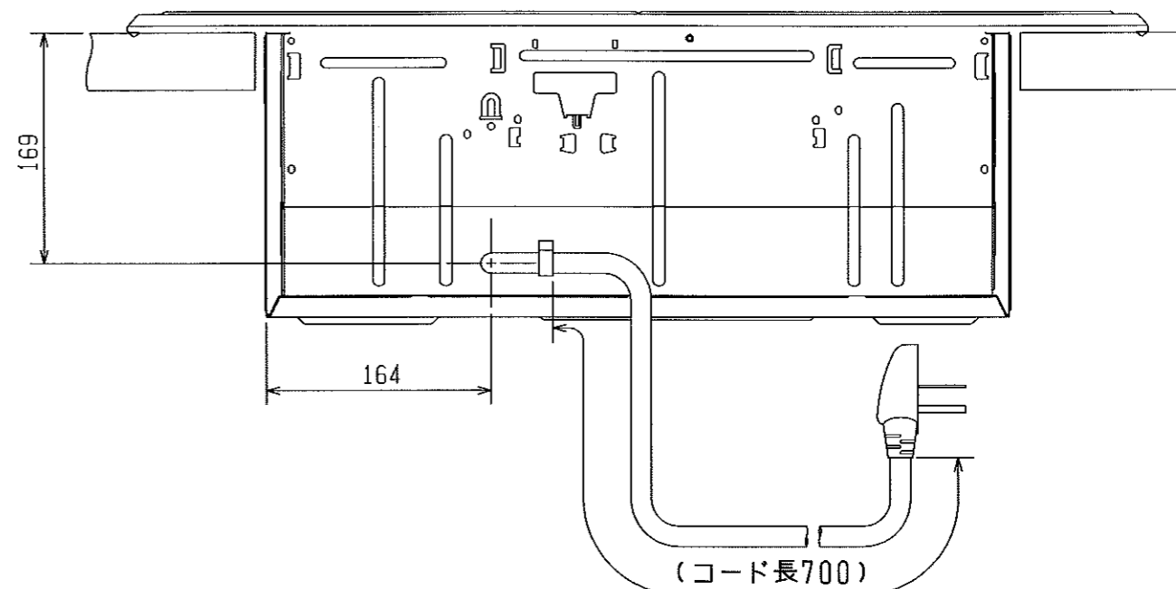
【背面図】
