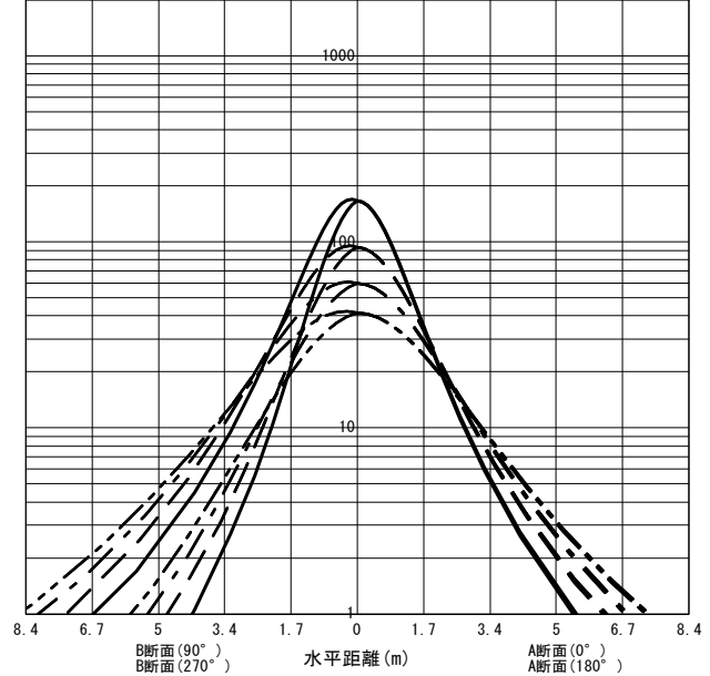
○直射水平面照度 (全光束: 1280 × 1 = 1280lm/台) 照度 (lx) — H1.50m --- H2.00m - - - H2.50m - · - · H3.00m (保守率: 1.00)
