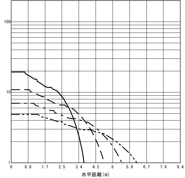
○直射水平面照度 (全光束: 352 × 1 = 352lm/台) 照度 (lx) — H1.50m --- H2.00m - - - H2.50m - · - · H3.00m (保守率: 1.00)
