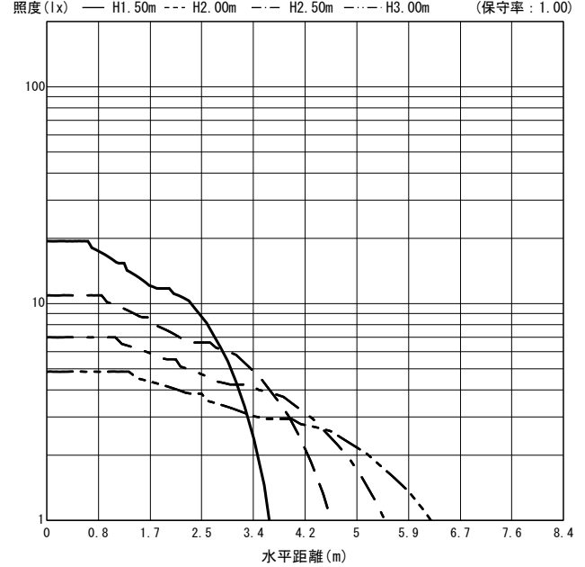
○直射水平面照度 (全光束: 352 × 1 = 352lm/台)
