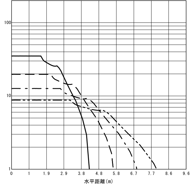
○直射水平面照度 (全光束 : 998 × 1 = 998lm/台) 照度 (lx) — H1.50m --- H2.00m - - - H2.50m - · - · H3.00m (保守率 : 1.00)
