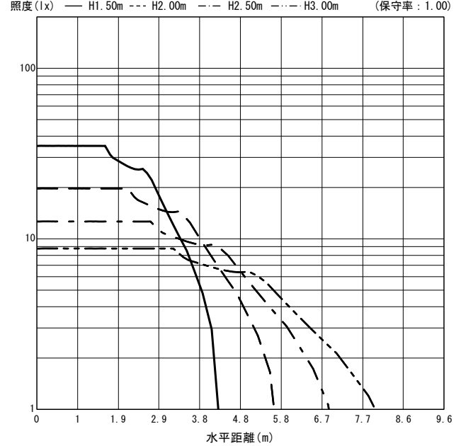
○直射水平面照度 (全光束 : 998 × 1 = 998lm/台)
