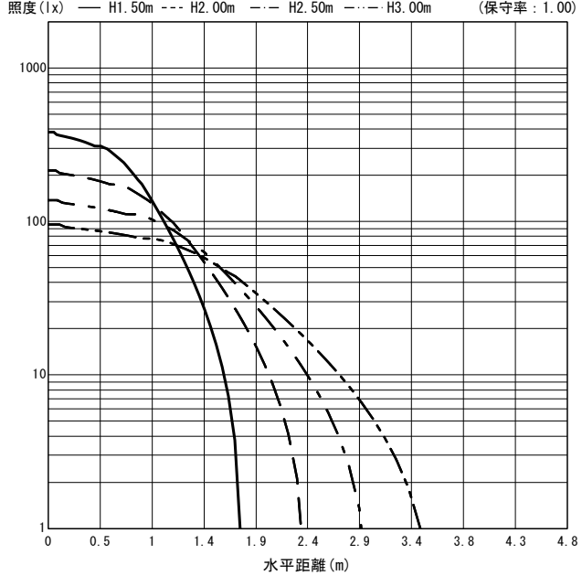
○直射水平面照度 (全光束: 1006 × 1 = 1006lm/台)
