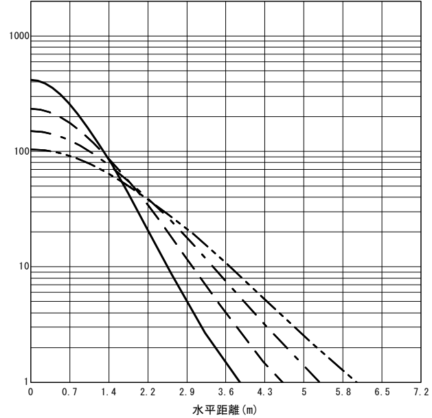
○直射水平面照度 (全光束: 1840 × 1 = 1840lm/台) 照度 (lx) — H1.50m --- H2.00m - - - H2.50m - · - · H3.00m (保守率: 1.00)
