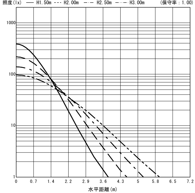
○直射水平面照度 (全光束: 1710 × 1 = 1710lm/台)
