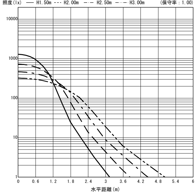
○直射水平面照度 (全光束: 3780 × 1 = 3780lm/台)
