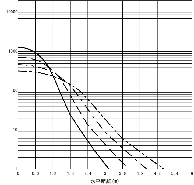
○直射水平面照度 (全光束: 3770 × 1 = 3770lm/台) 照度 (lx) — H1.50m --- H2.00m - - - H2.50m - · - · H3.00m (保守率: 1.00)
