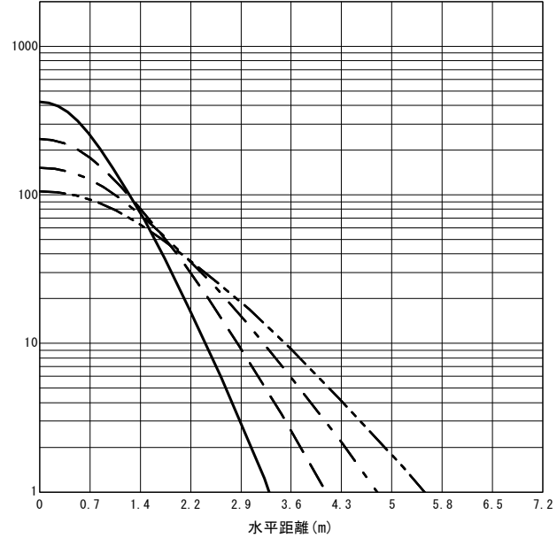
○直射水平面照度 (全光束: 1650 × 1 = 1650lm/台) 照度 (lx) — H1.50m --- H2.00m - - - H2.50m - · - · H3.00m (保守率: 1.00)
