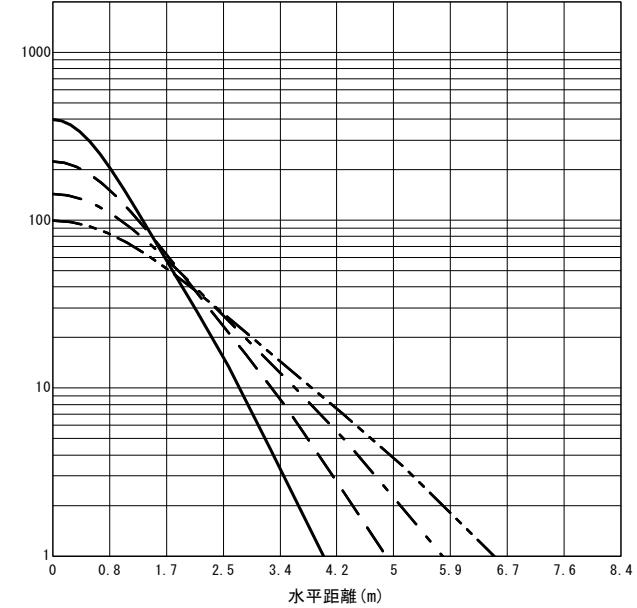
○直射水平面照度 (全光束: 1890 × 1 = 1890lm/台) 照度 (lx) — H1.50m --- H2.00m - - - H2.50m - · - · H3.00m (保守率: 1.00)
