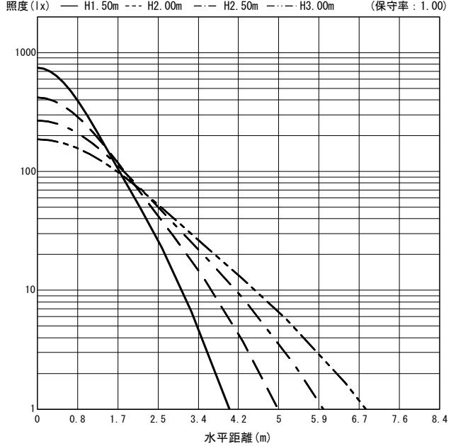
○直射水平面照度 (全光束: 3460 × 1 = 3460lm/台)
