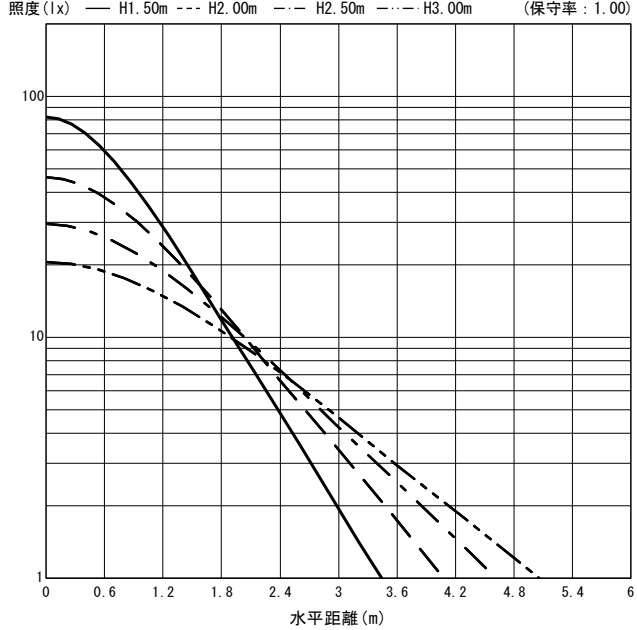
○直射水平面照度 (全光束: 450 × 1 = 450lm/台)
