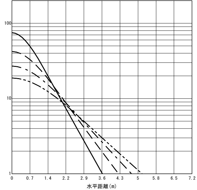
○直射水平面照度 (全光束: 450 × 1 = 450lm/台) 照度 (lx) — H1.50m --- H2.00m - - - H2.50m - · - · H3.00m (保守率: 1.00)
