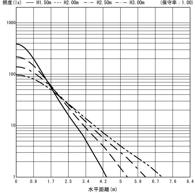
○直射水平面照度 (全光束: 1890 × 1 = 1890lm/台)
