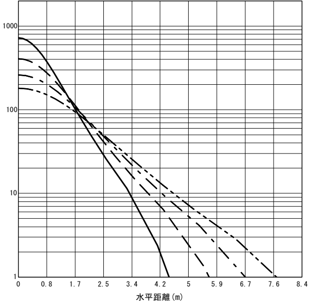
○直射水平面照度 (全光束 : 3490 × 1 = 3490lm/台) 照度 (lx) — H1.50m --- H2.00m - - - H2.50m - · - · H3.00m (保守率 : 1.00)
