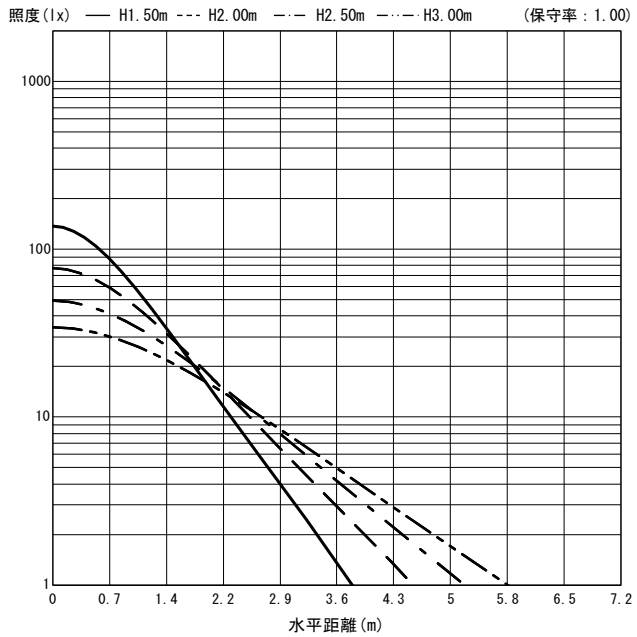
○直射水平面照度 (全光束 : 755 × 1 = 755lm/台)
