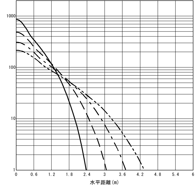
○直射水平面照度 (全光束: 1660 × 1 = 1660lm/台) 照度 (lx) — H1.50m --- H2.00m - - - H2.50m - · - · H3.00m (保守率: 1.00)
