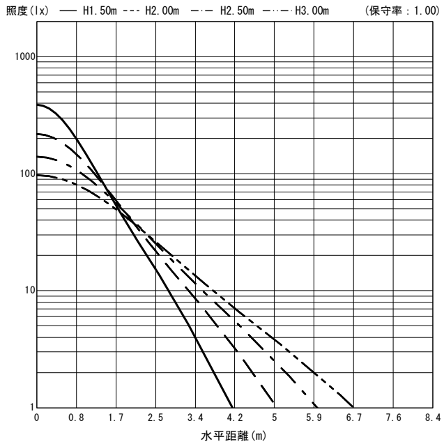
○直射水平面照度 (全光束: 1830 × 1 = 1830lm/台)
