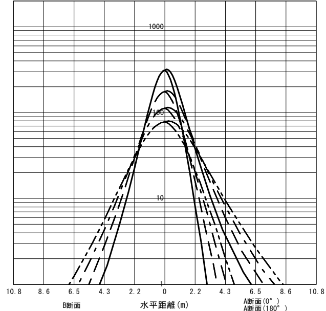
○直射水平面照度 (全光束: 1530 × 1 = 1530lm/台) 照度 (lx) — H1.50m --- H2.00m - - - H2.50m - · - · H3.00m (保守率: 1.00)
