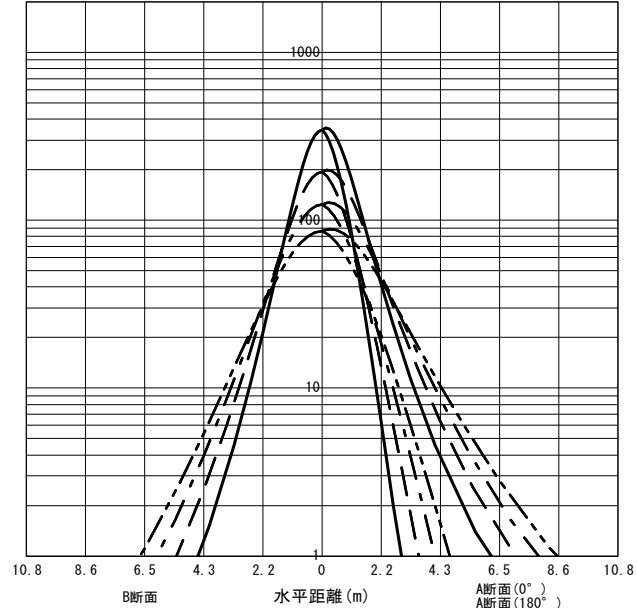
○直射水平面照度 (全光束: 1730 × 1 = 1730lm/台) 照度 (lx) — H1.50m --- H2.00m - - - H2.50m - · - · H3.00m (保守率: 1.00)
