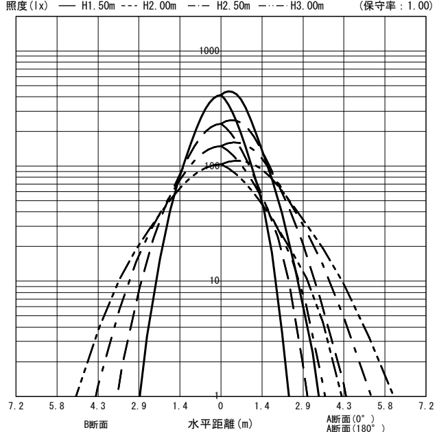
○直射水平面照度 (全光束: 1770 × 1 = 1770lm/台)
