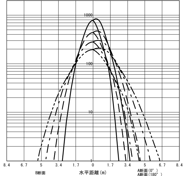
○直射水平面照度 (全光束: 3340 × 1 = 3340lm/台) 照度 (lx) — H1.50m --- H2.00m - - - H2.50m - · - · H3.00m (保守率: 1.00)
