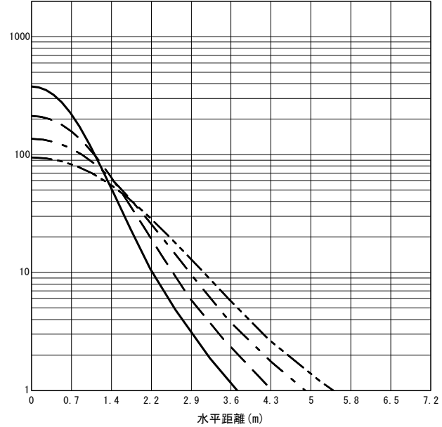
○直射水平面照度 (全光束: 1350 × 1 = 1350lm/台) 照度 (lx) — H1.50m --- H2.00m - - - H2.50m - · - · H3.00m (保守率: 1.00)
