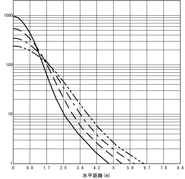
○直射水平面照度 (全光束: 3240 × 1 = 3240lm/台) 照度 (lx) — H1.50m --- H2.00m - - - H2.50m - · - · H3.00m (保守率: 1.00)
