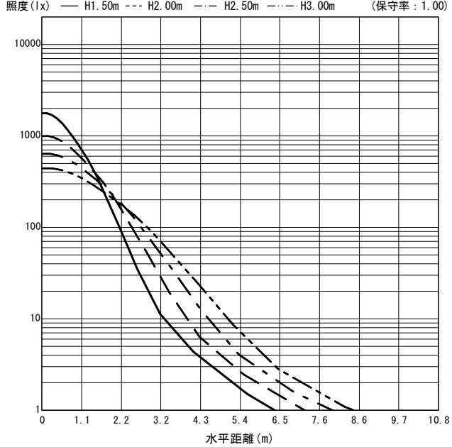
○直射水平面照度 (全光束: 8320 × 1 = 8320lm/台)
