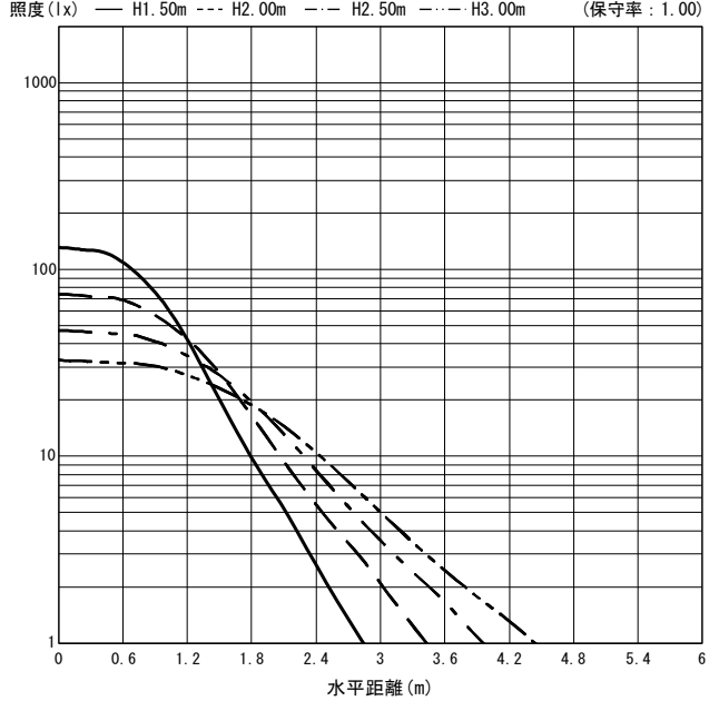
○直射水平面照度 (全光束 : 570 × 1 = 570lm/台)
