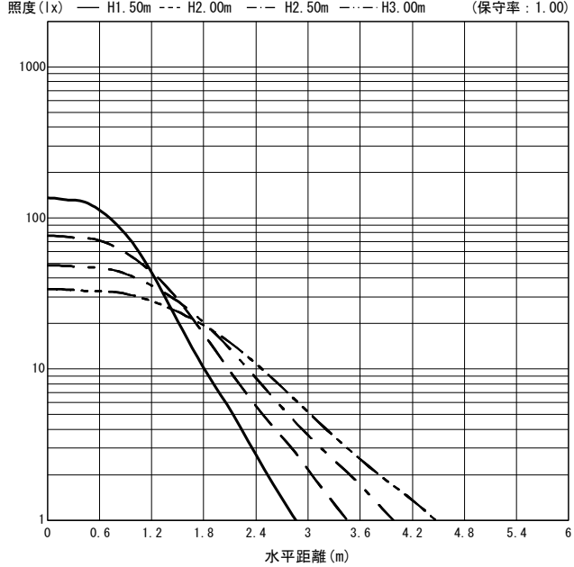
○直射水平面照度 (全光束 : 590 × 1 = 590lm/台)
