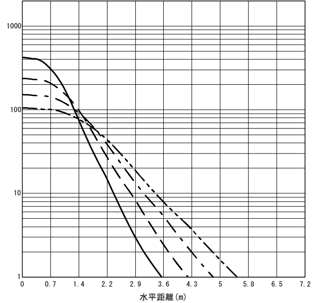
○直射水平面照度 (全光束: 1830 × 1 = 1830lm/台) 照度 (lx) — H1.50m --- H2.00m - - - H2.50m - · - · H3.00m (保守率: 1.00)
