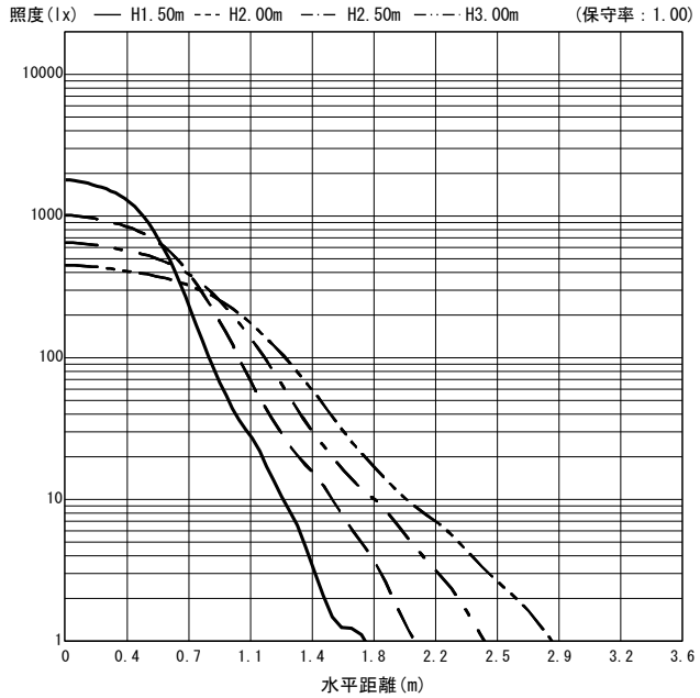
○直射水平面照度 (全光束: 1660 × 1 = 1660lm/台)
