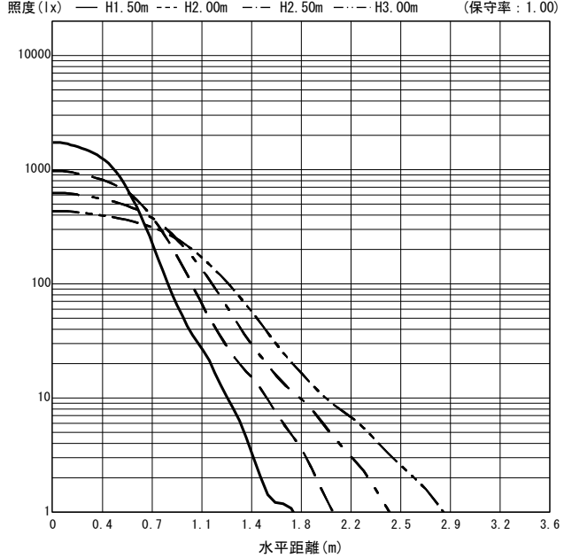
○直射水平面照度 (全光束: 1610 × 1 = 1610lm/台)
