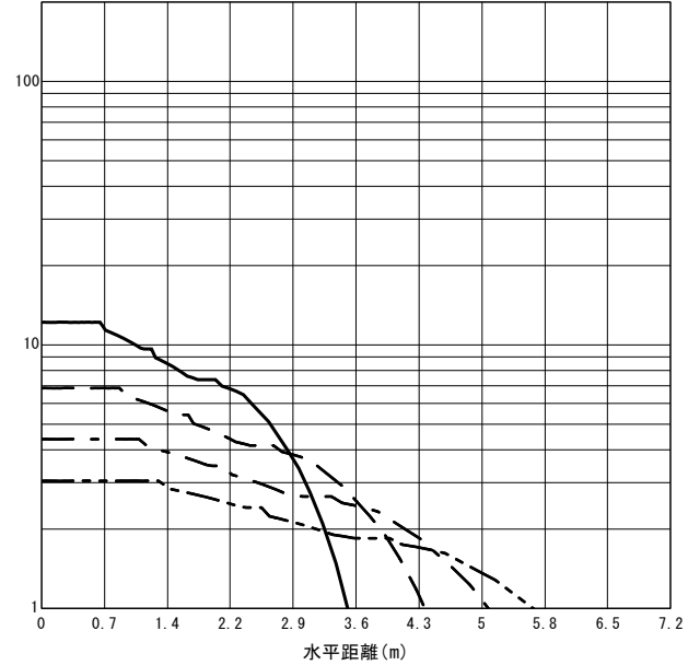
○直射水平面照度 (全光束 : 221 × 1 = 221lm/台) 照度 (lx) — H1.50m --- H2.00m - - - H2.50m - · - · H3.00m (保守率 : 1.00)
