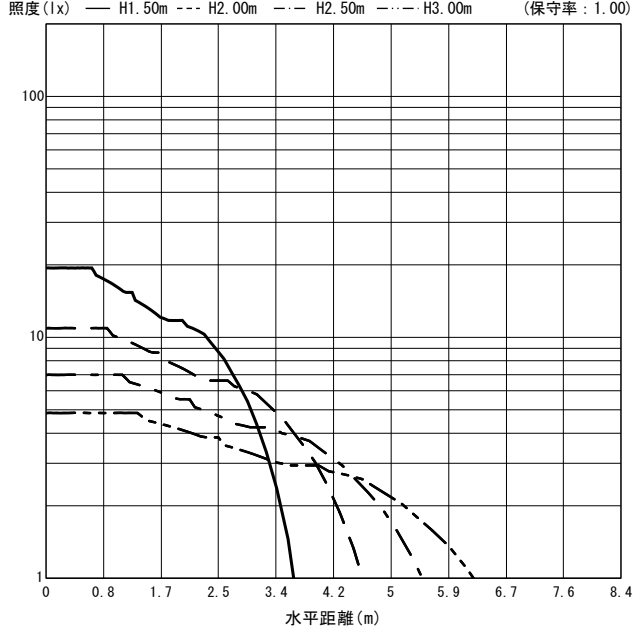
○直射水平面照度 (全光束: 352 × 1 = 352lm/台)
