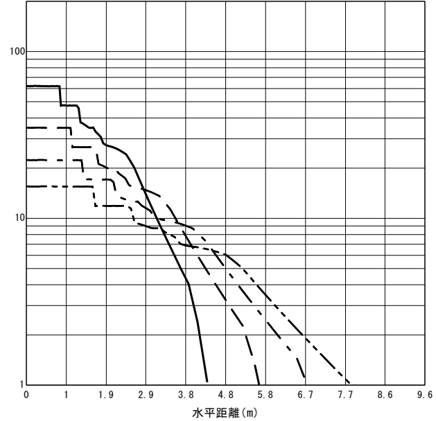
○直射水平面照度 (全光束: 1005 × 1 = 1005lm/台) 照度 (lx) — H1.50m --- H2.00m - - - H2.50m - · - · H3.00m (保守率: 1.00)
