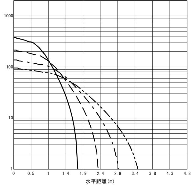
○直射水平面照度 (全光束：1006 × 1 = 1006lm/台) 照度 (lx) — H1.50m --- H2.00m - - - H2.50m - · - · H3.00m (保守率：1.00)
