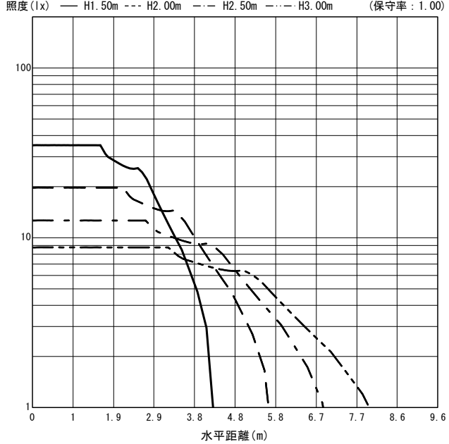
○直射水平面照度 (全光束 : 998 × 1 = 998lm/台)
