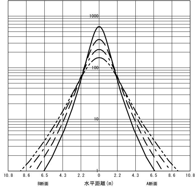
○直射水平面照度 (全光束: 3880 × 1 = 3880lm/台) 照度 (lx) — H1.50m --- H2.00m - - - H2.50m - · - · H3.00m (保守率: 1.00)
