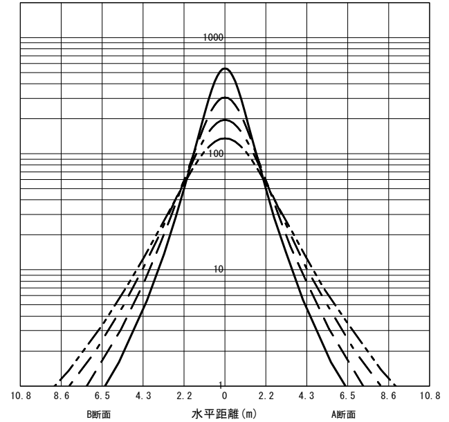
○直射水平面照度 (全光束: 3360 × 1 = 3360lm/台) 照度 (lx) — H1.50m --- H2.00m - - - H2.50m - · - · H3.00m (保守率: 1.00)
